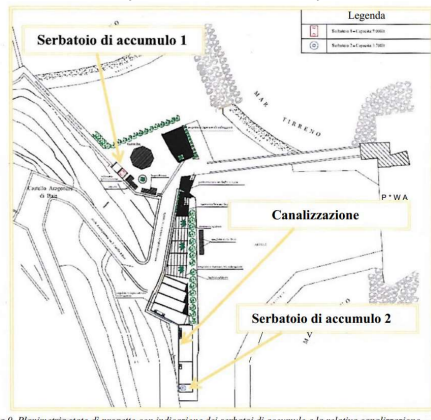
Figura 9. Planimetria stato di progetto con indicazione dei serbatoi di accumulo e la relativa canalizzazione.
